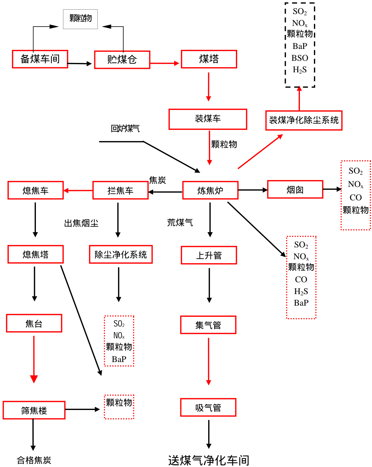
附图 1 炼焦及焦处理工艺流程排污环节示意图
