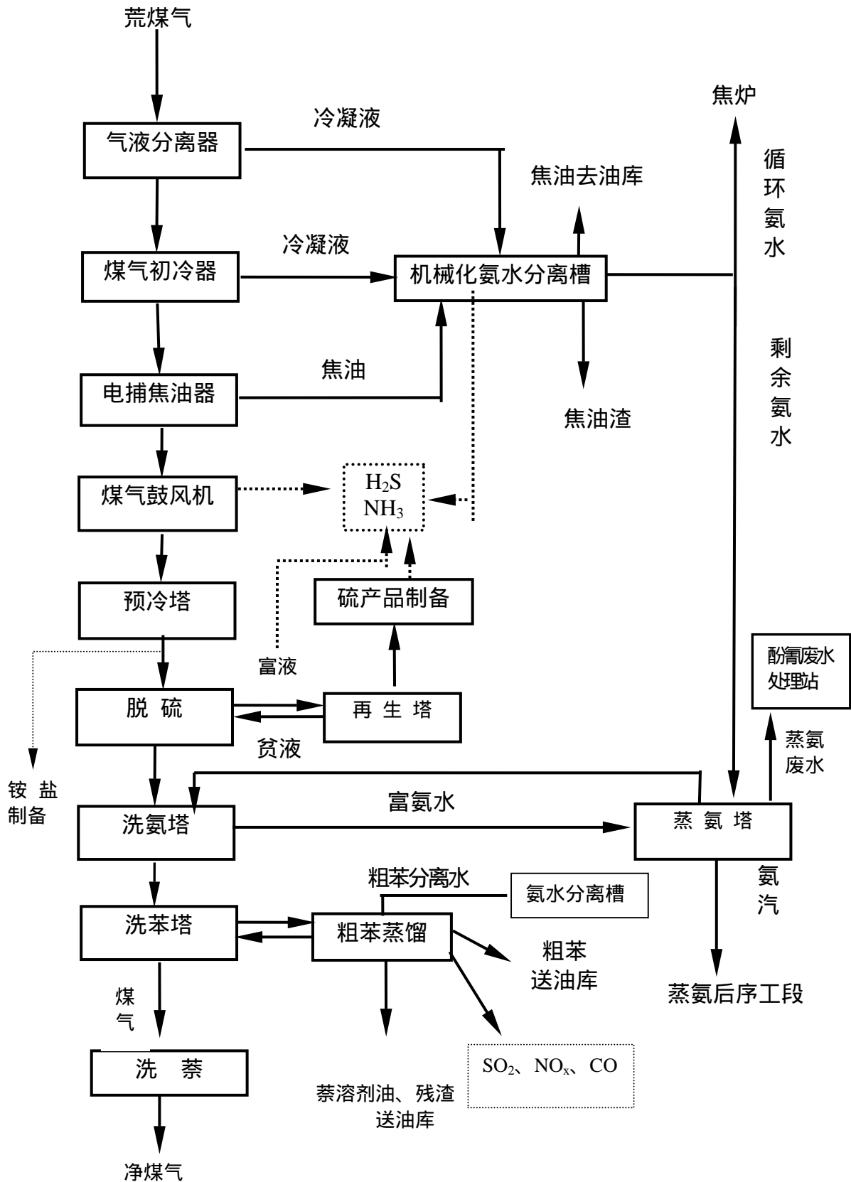
附图2 煤气净化车间工艺及排污流程图
